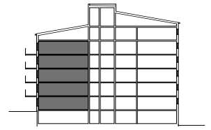
SEKTION
